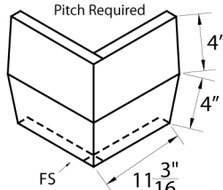
Gutter End Cap
